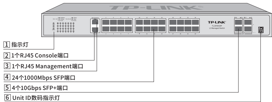
图1-2 TL-SH6428F前面板示意图
