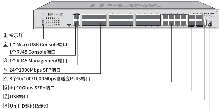
图1-4 TL-SH7428F前面板示意图
